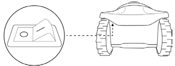
Sicherheitsschalter
